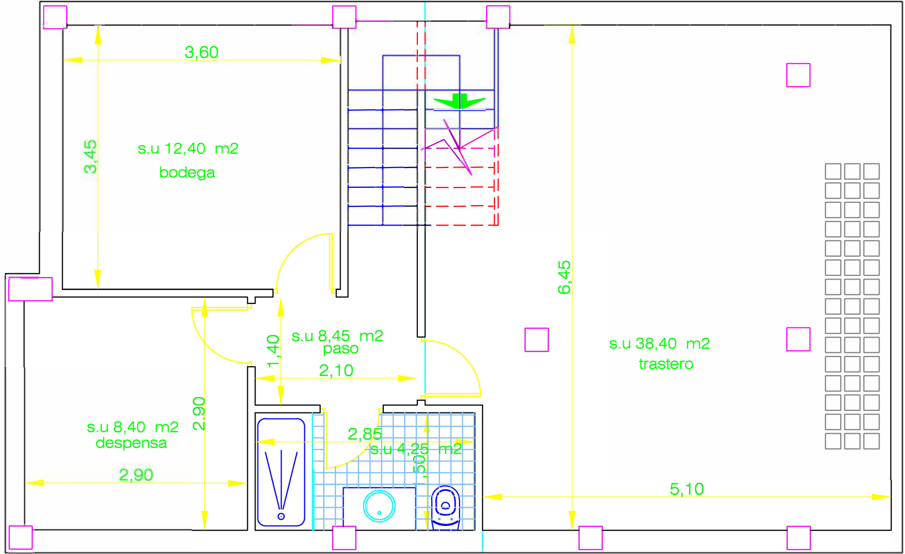
PLANTA SOTANO
