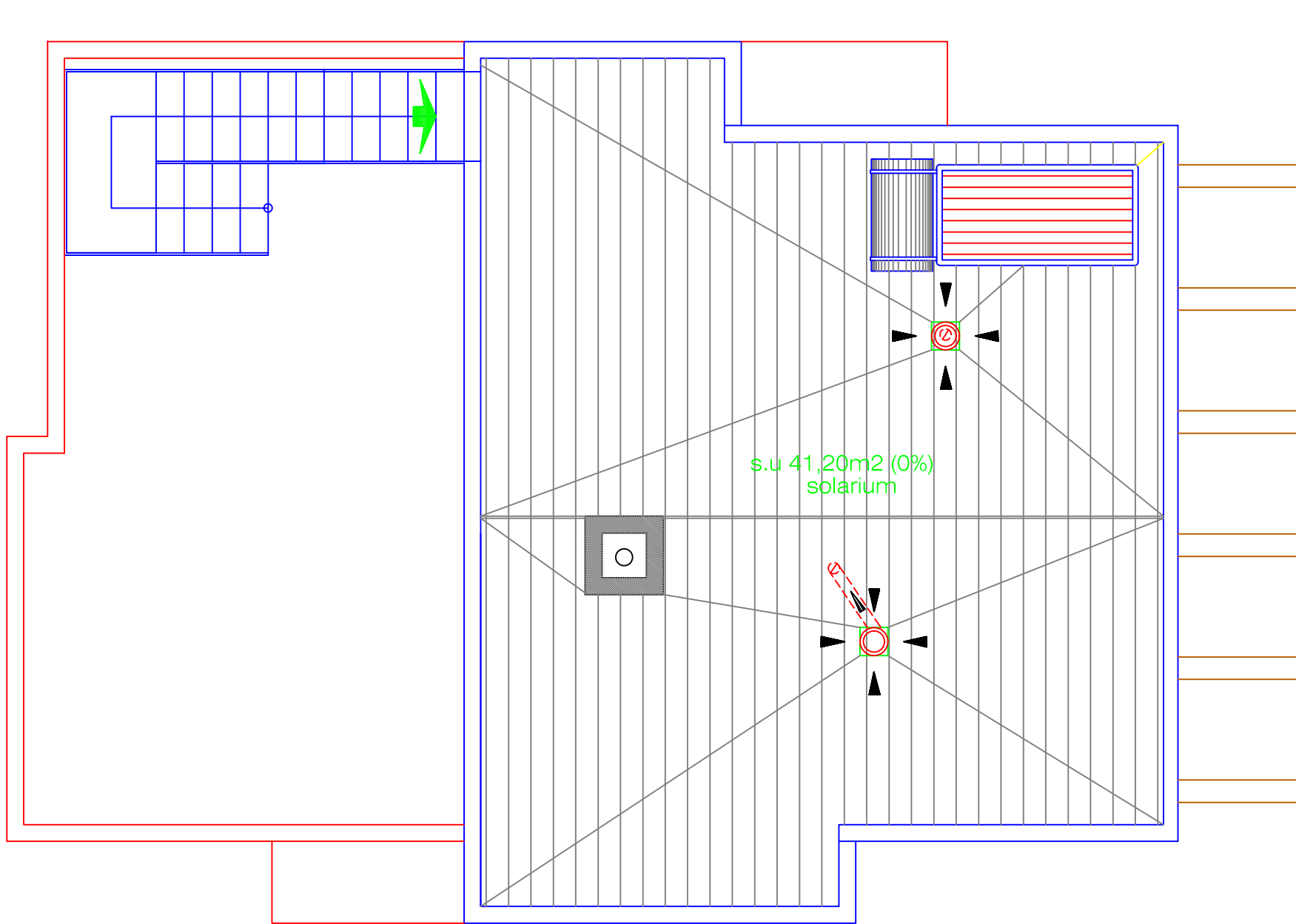
PLANTA SOLARIUM
